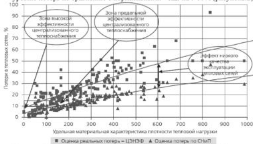
Рис. 2.2. Зависимость потерь в тепловых сетях от удельной материальной характеристики тепловых сетей
