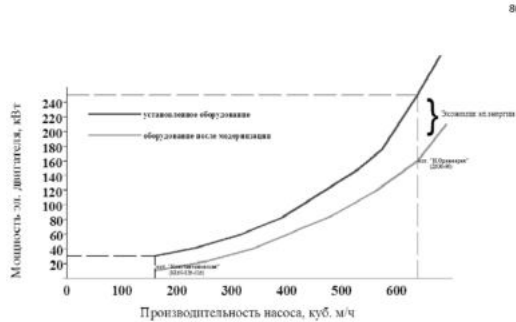
Рис.5.6. Зависимость мощности электродвигателя привода насоса от его производительности
