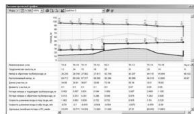
Рис.13.13. Пьезометрический график
