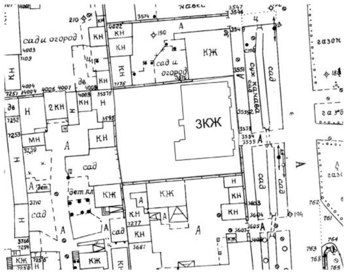
Ситуационный план земельного участка М 1:500
